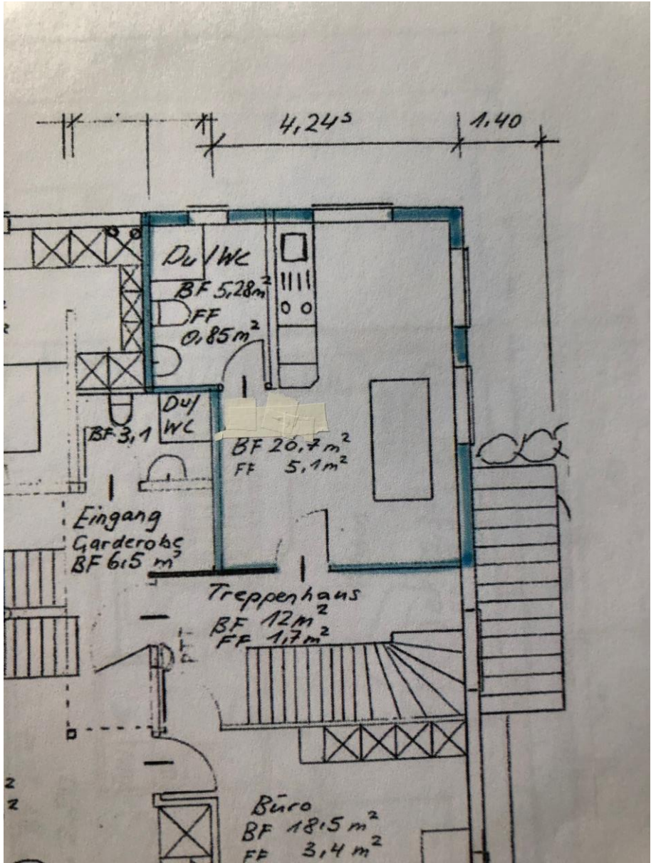
Grundriss
